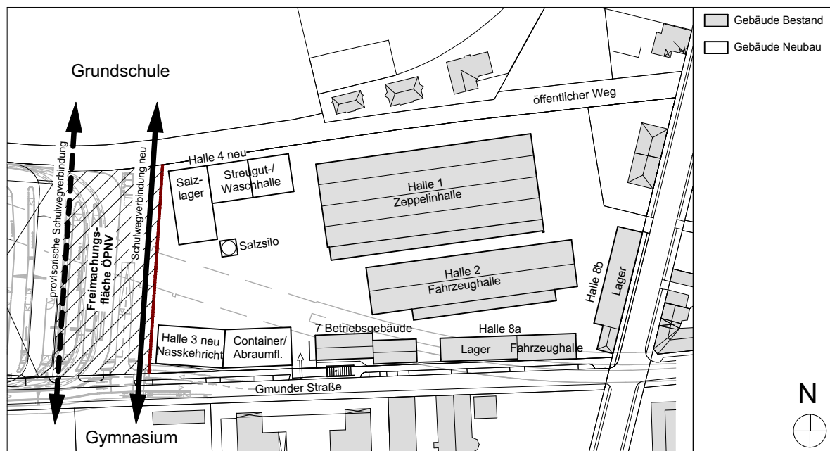
Lageplan Neubau, Schulwegeverbindung
