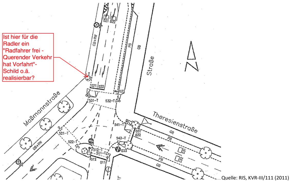
Planauszug Kreuzung Schleißheimer-/ Theresien-/ Maßmannstraße
